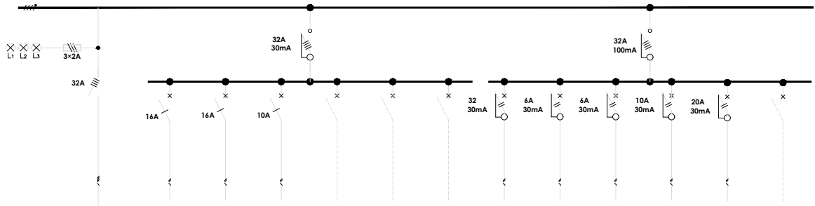
QUADRO DA REFEITORIO (Q_PS5) Normal L1,L2,L3,N,PE AC 230/400 V
